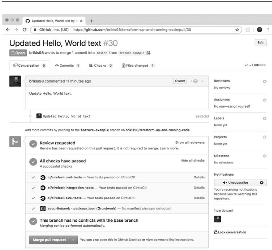
Рис. 8.2. В запросе на включение внесенных изменений в GitHub показываются результаты автоматических тестов из CircleCI
