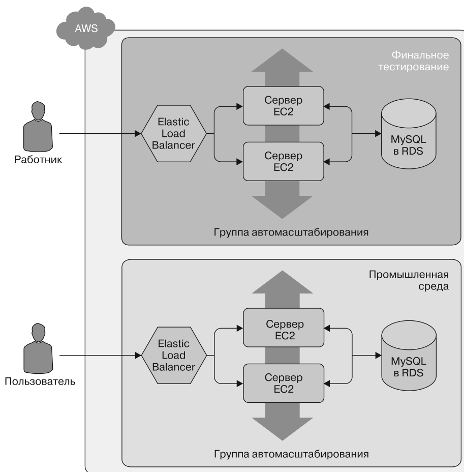
Рис. 4.2. Две среды, каждая со своим балансировщиком нагрузки, кластером веб-серверов и базой данных
