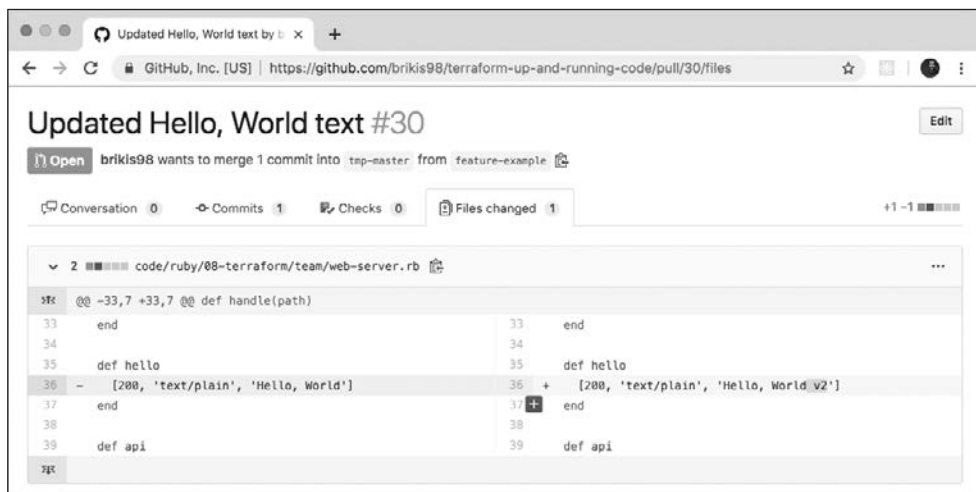
Рис. 8.1. Запрос на включение внесенных изменений в GitHub
