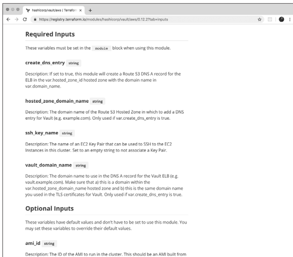
Рис. 6.5. Реестр Terraform автоматически анализирует и отображает ввод и вывод модуля
