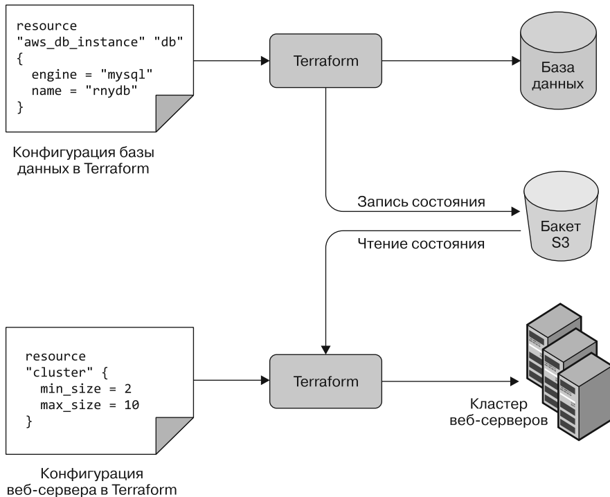
Рис. 3.11. База данных записывает свое состояние в бакет S3 ( вверху ), а кластер веб-серверов считывает его из того же бакета ( внизу )
