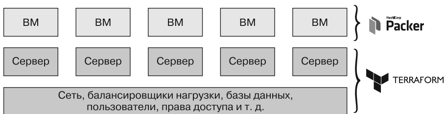
Рис. 1.10. Совместное применение Terraform и Packer
