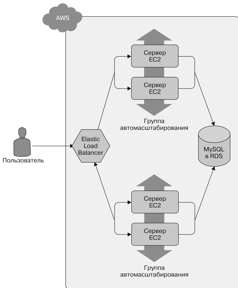
Рис. 5.4. Серверы в новой группе ASG загрузились, подключились к БД, зарегистрировались в ALB и начали обслуживать запросы
