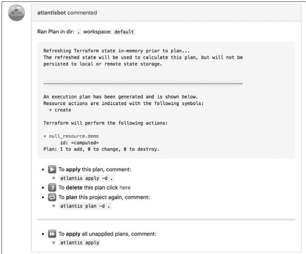
Рис. 8.3. Atlantis умеет автоматически добавлять вывод команды terraform plan в виде комментариев к запросам на включение внесенных изменений
