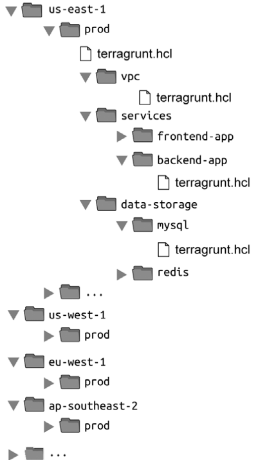
Рис. 8.5. Структура файлов и каталогов при использовании Terragrunt
