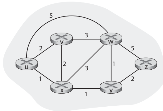
Рис. 4.27. Абстрактная модель компьютерной сети в виде графа
