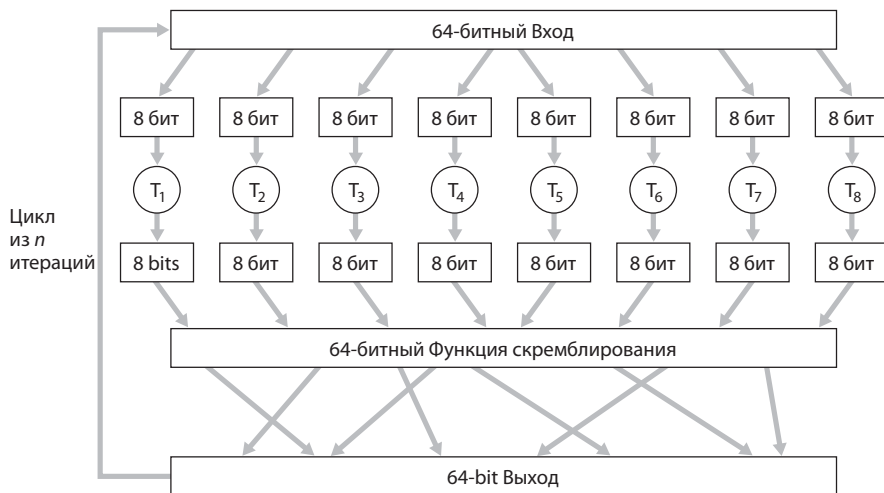
Рис. 8.5. Пример блочного шифра
