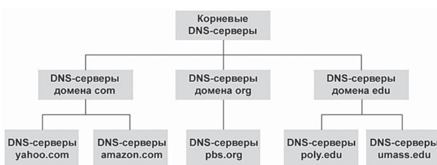
Рис. 2.19. Часть иерархической структуры DNS-серверов
