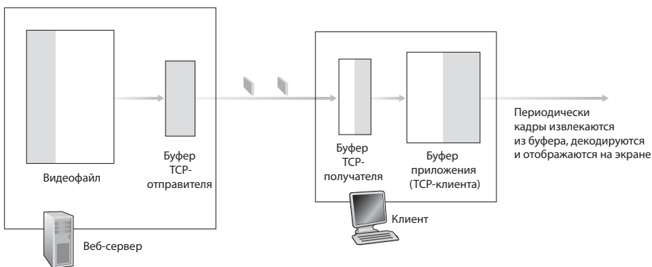
Рис. 7.2. Потокное вещание статического видео по протоколам HTTP/TCP
