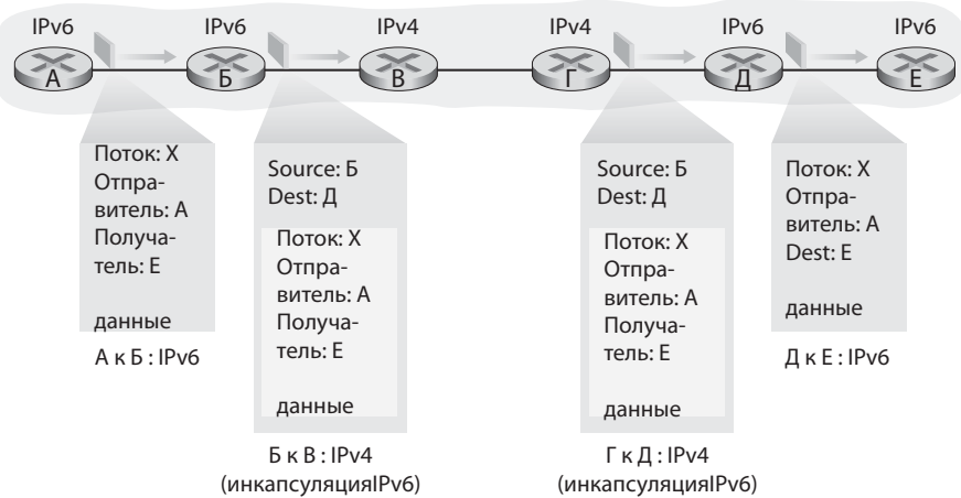
Рис. 4.26. Туннелирование
