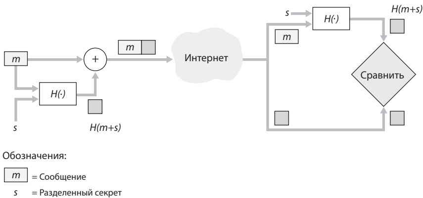
Рис. 8.9. Код аутентификации сообщения (MAC)
