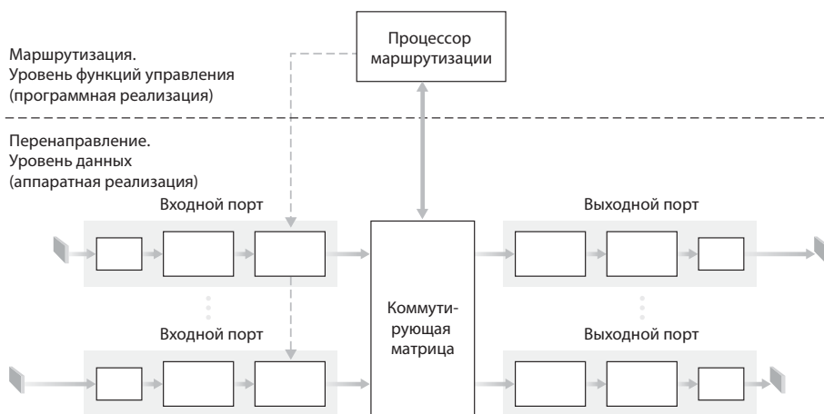
Рис. 4.6. Архитектура маршрутизатора
