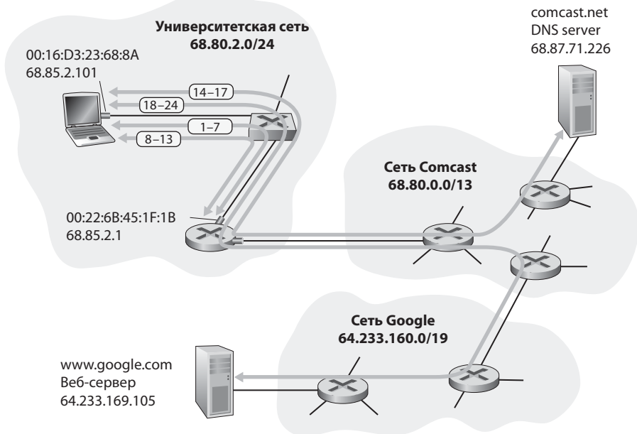
Рис. 5.32. Один день из жизни запроса веб-страницы. Схема сети и действия в ней
