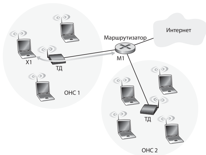
Рис. 6.14. Использование полей адреса в кадрах данных 802.11: пересылка кадров между X1 и M1
