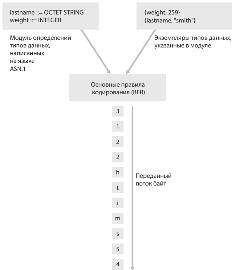
Рис. 9.9. Пример кодирования в системе BER
