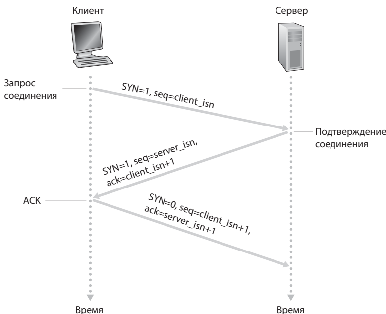
Рис. 3.39. Обмен сегментами в тройном рукопожатии протокола ТСР
