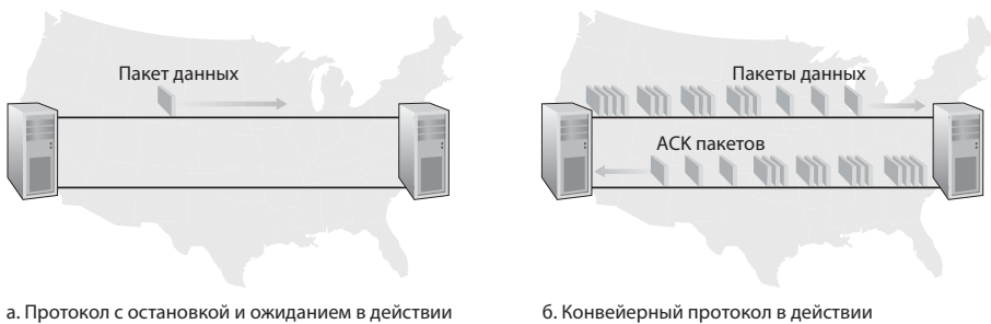
Рис. 3.17. Версия протокола с ожиданием подтверждений и с конвейеризацией
