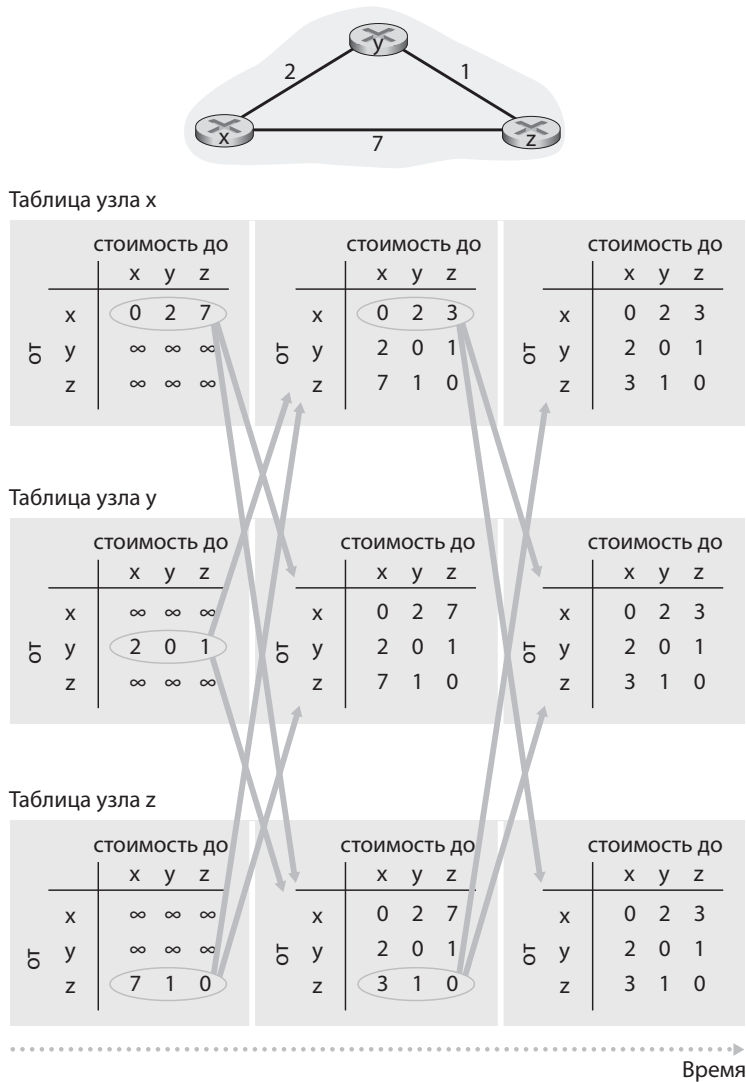
Рис. 4.30. Дистанционно-векторный алгоритм
