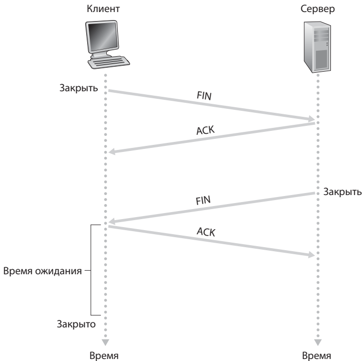
Рис. 3.40. Завершение TCP-соединения
