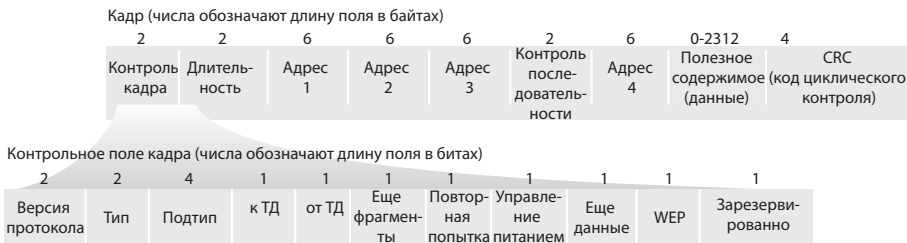
Рис. 6.13. Кадр 802.11
