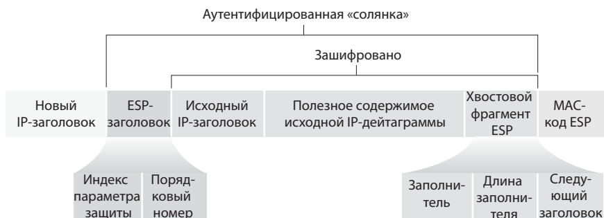
Рис. 8.29. Формат IPsec-дейтаграммы
