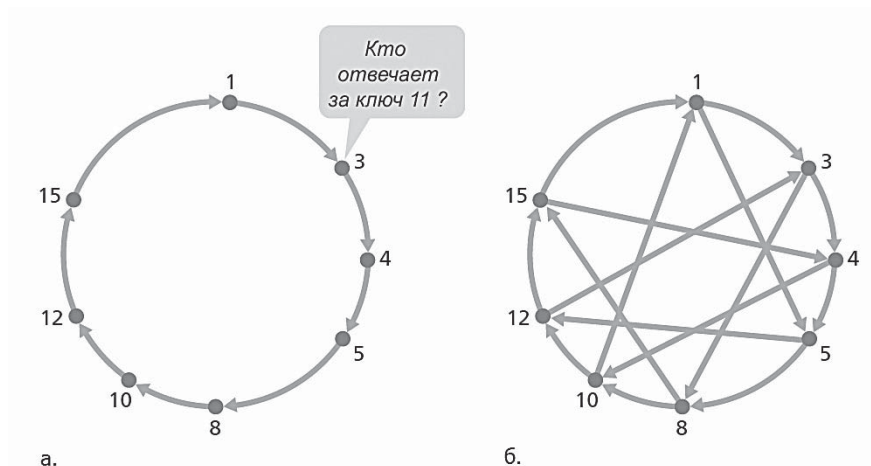
Рис. 2.27 (а). Циркулярная распределенная хеш-таблица. Пир 3 пытается определить, кто отвечает за ключ 11. (б). Циркулярная таблица со ссылками
